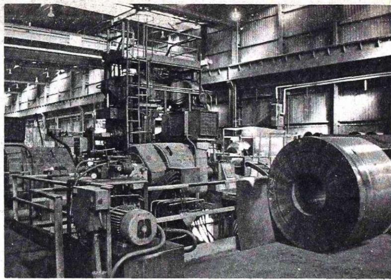
Dresirno ogrodje v Hladni valjarni Bela (foto: Irena Kučina)
