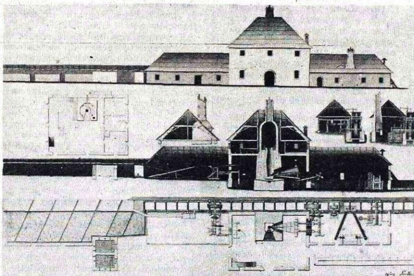
Originalen načrt znamenitega Zoisovega plavža na Javorniku iz leta 1797
