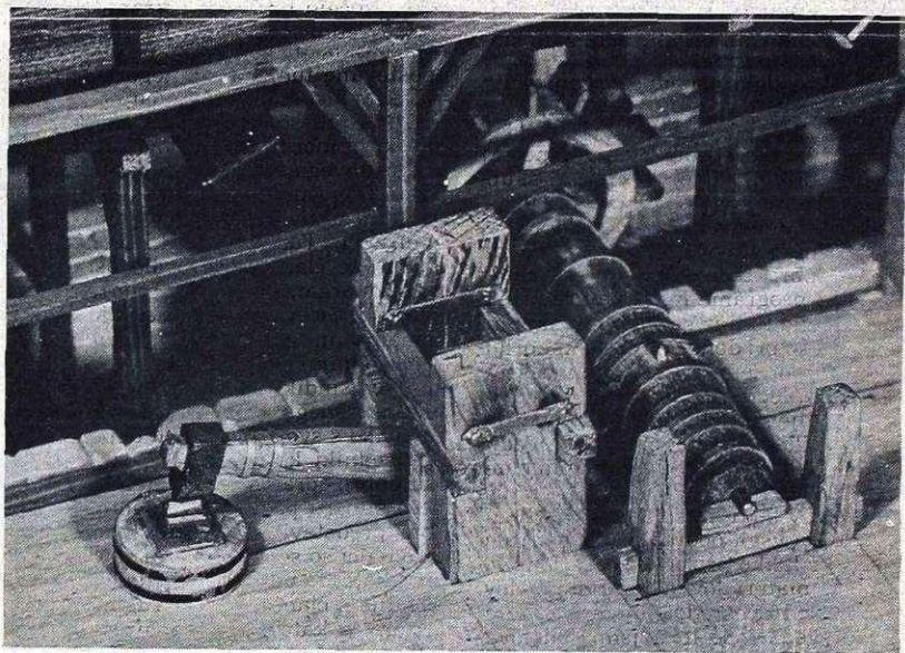
Maketa kovačnice z »norcem« (fotoarhiv Tehniškega muzeja)
