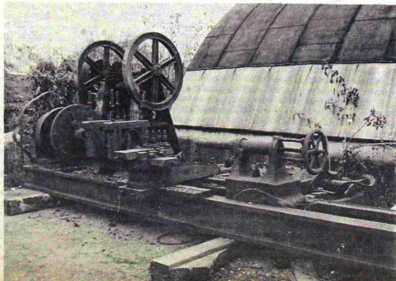
Najstarejša ohranjena stružnica Kōrosi iz leta 1861 (foto: Silvo Kokalj)
