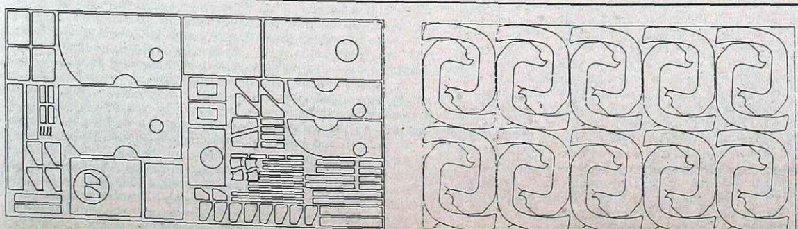
Primer krojene pločevine
