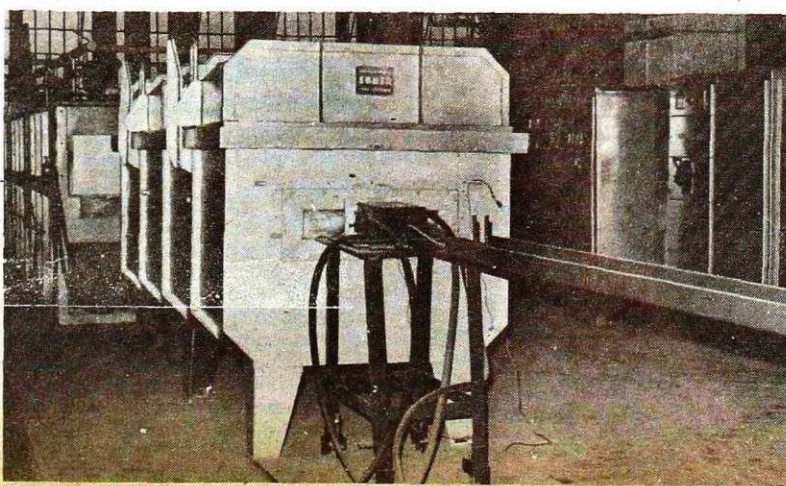
Pilotna naprava za kaljenje hladno valjanih trakov (foto: Irena Kučina)
