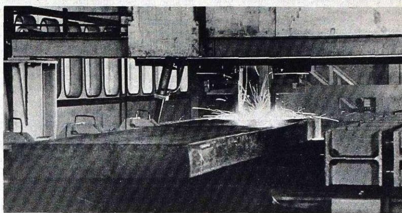
Linija za razrez slabov (foto: I. Kučina)
