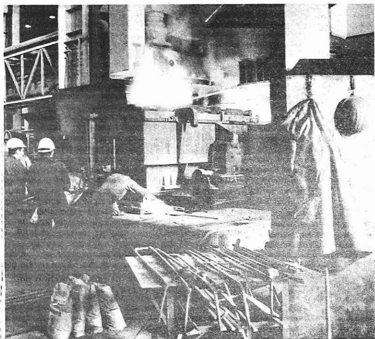
Na kontilivu v Jeklarni 2 (foto: Irena Kučina)
