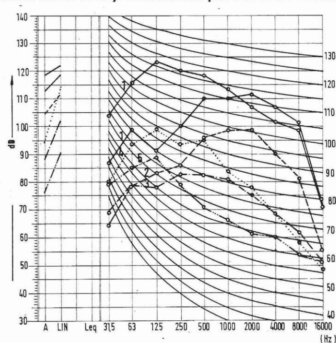
Učinek zvočne izolacije elektroobločne peči s komoro v Jeklarni 2
