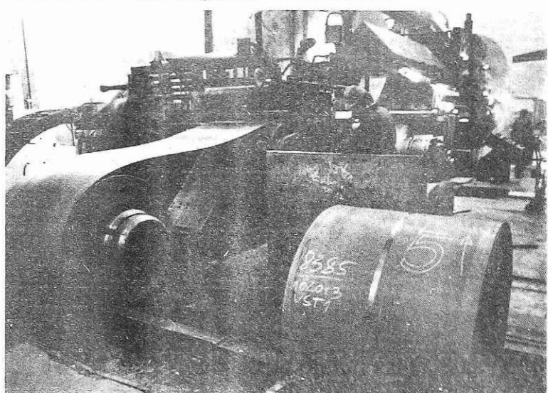
Sendzimir ogrodje v Hladni valjarni Bela (foto: Irena Kučina)
