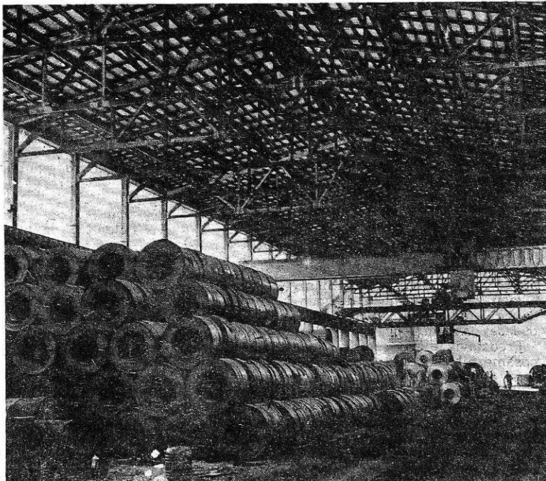
V Hladni valjarni Jesenice (foto: I. Kučina)
