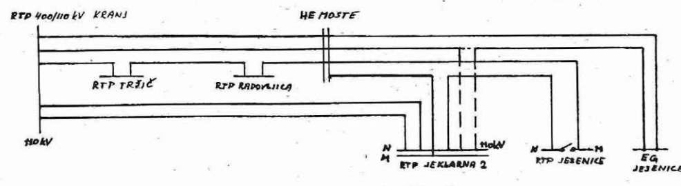
110 kV omrežje od RTP 400/110 kV Kranj do Jesenic (slika 8)
