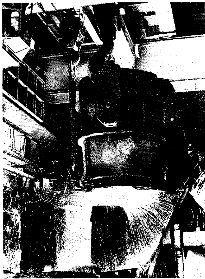
Vlivanje jekla v kokile (foto: I. Kučina)
