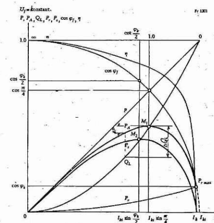
Karakteristike peči U_f : napetost peči P : navidezna moč
