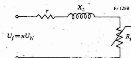
Slika 2 Nadomestna shema ene faze peči.
