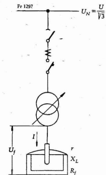
Slika 1 Enopolna shema trifazne peči
