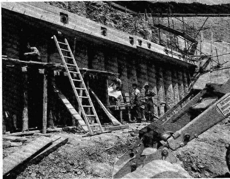
Gradnja karavanškega predora (foto I. Kučina)
