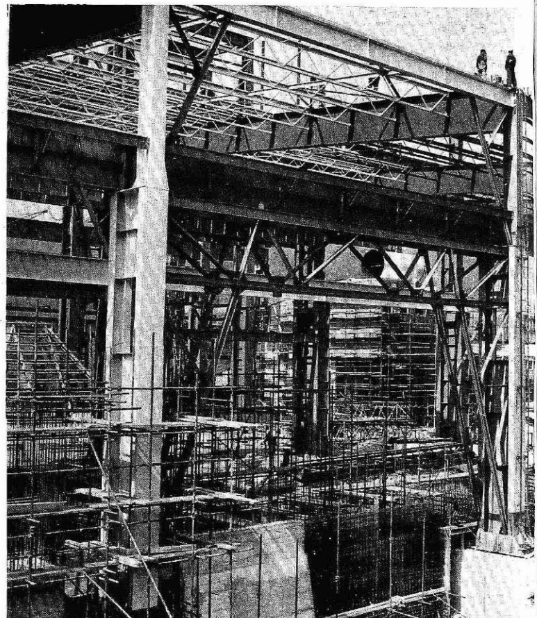
Gradnja Jeklarne 2 (foto I. Kučina)
