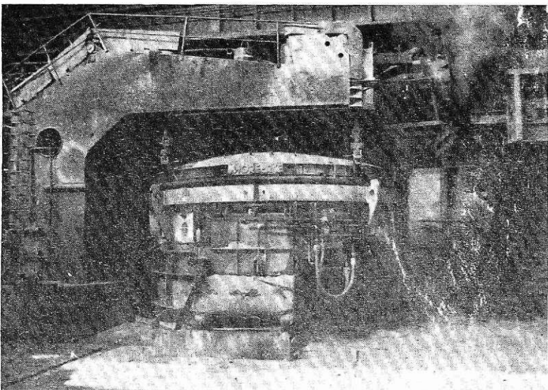
Remont elektro peči ASEA (S. Kokalj)
