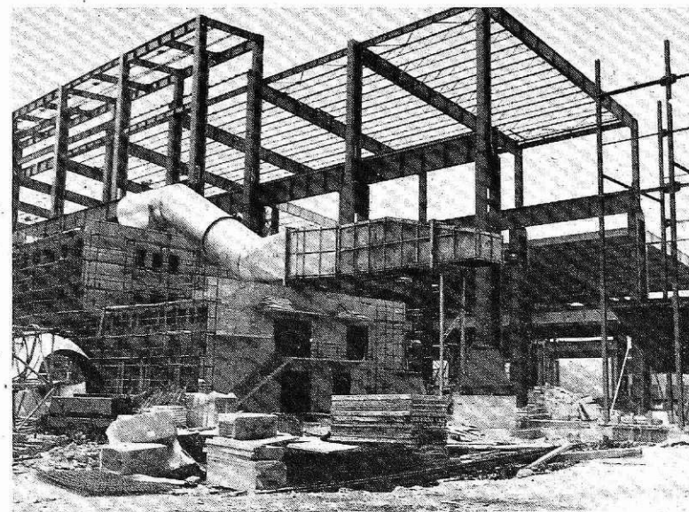
Gradnja Jeklarne 2 (foto I. Kučina)
