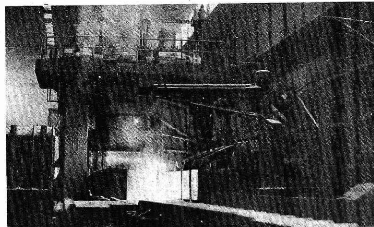
V Valjarni bluming (foto I. Kučina)
