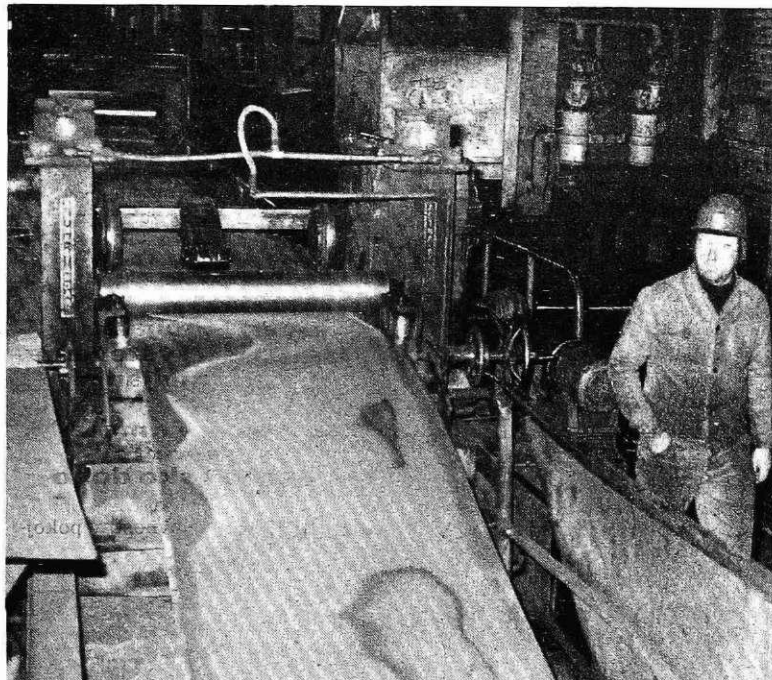
V adjuštaži bluminga (foto S. Kokalj)
