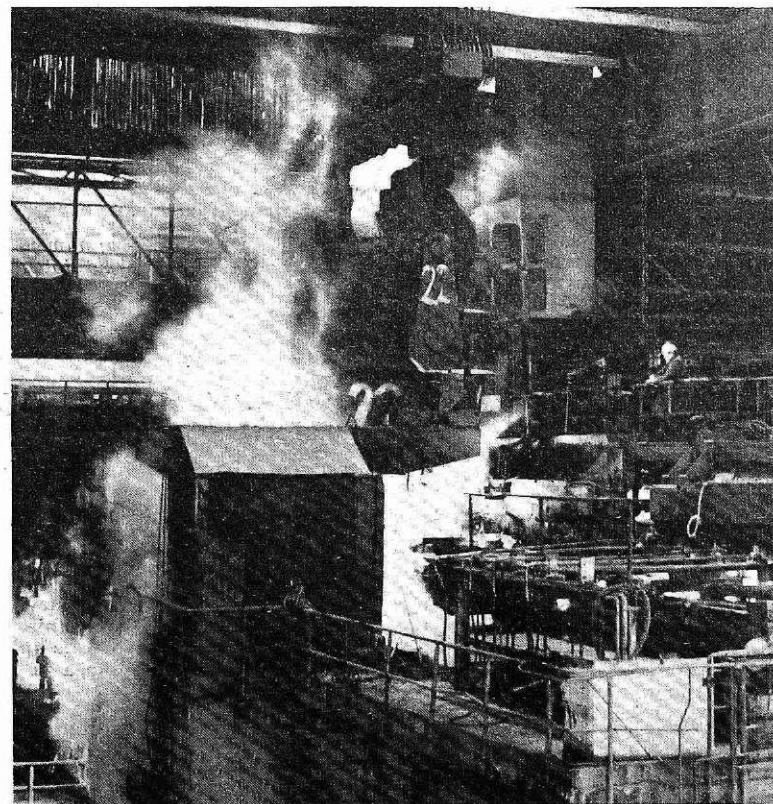
Vlivanje v kontilivu (foto I. Kučina)
