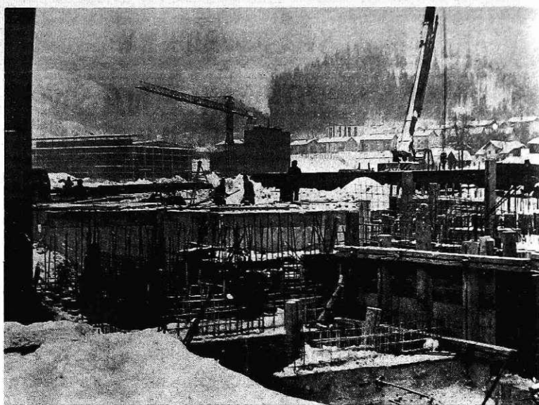
Jeklarna 2 (foto I. Kučina)
