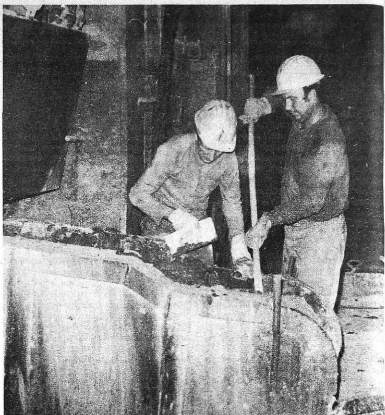
Obzidava livnega žleba martinovke (foto I. Kučina)
