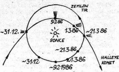
Slika 4: slika ponazarja zemljin tir in delira Halleyevega komet v bližini sonca. Datumi prikazujejo lego komet in zemlje ob istem dnevu (približno)
