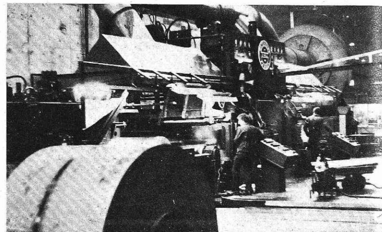
Senzimir ogrodje v HVB (foto I. Kučina)
