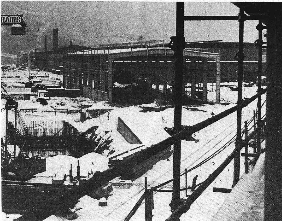
Gradbišče Jeklarnе 2 v teh dneh (foto I. Kučina)
