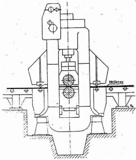
Valjarsko ogrodje — prerez
