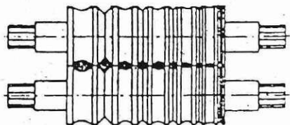
Kalibrirna valja za valjanje eliptičnega in kvadratnega profila
