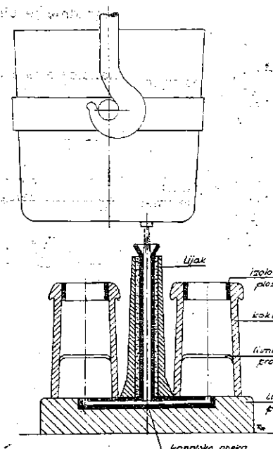
Vilvanje jekla iz livne ponve v kokile
