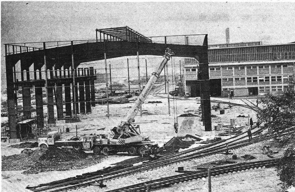
Konstrukcija (foto B. Grce)
