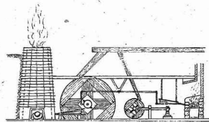
Fužine, kakršne najdemo po Evropi po letu 1000: meh za plavž in kovačnico poganja voda.
