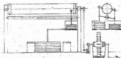
Vigenjska naprava na sapo: vodno kolo z ročico, navpično kozel, prečno samopih in levo pomožni samopih z berglo. Od cilindričnega mehova gre sapa po cevi v ješo.
