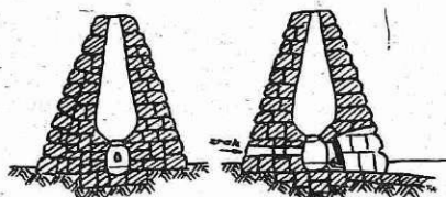
Preprosta visoka peč — prerez
