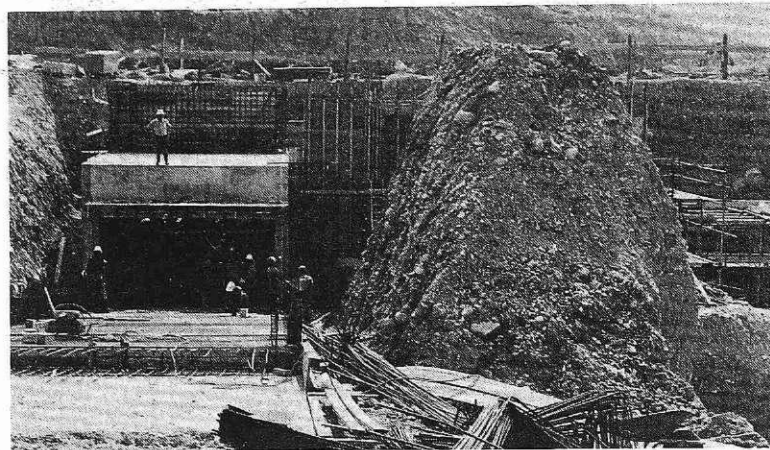
Razkladalna postaja s podzemnimi kanali (foto I. Kučina)
