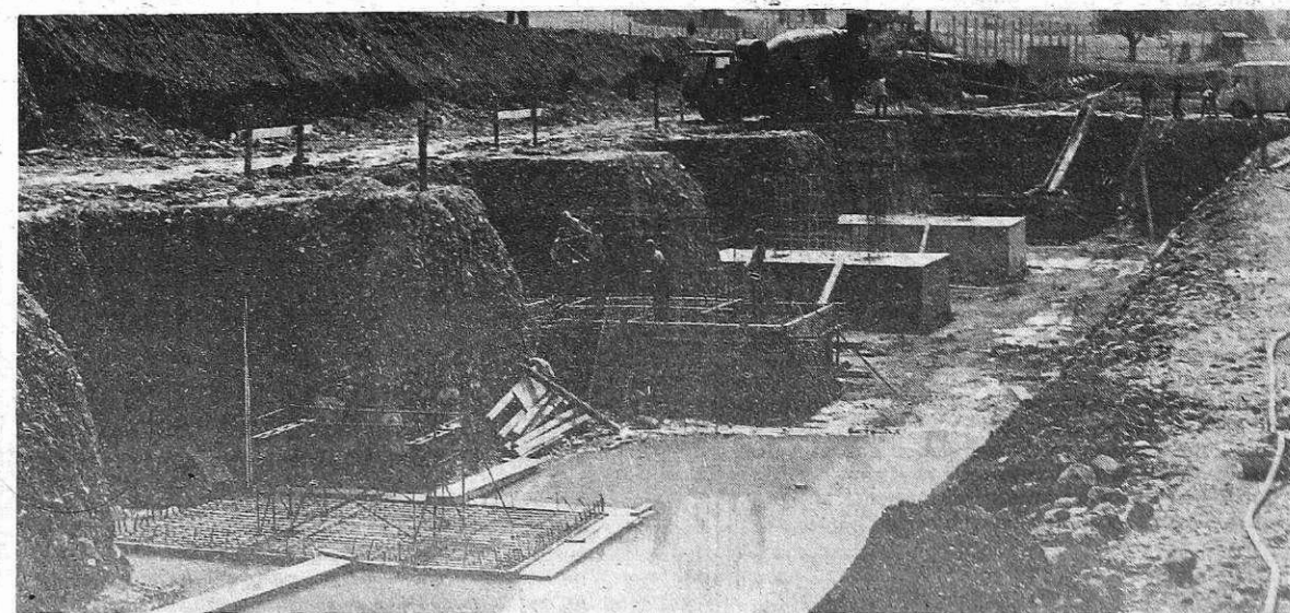
Gradnja jeklarne 2 (foto I. Kučina)
