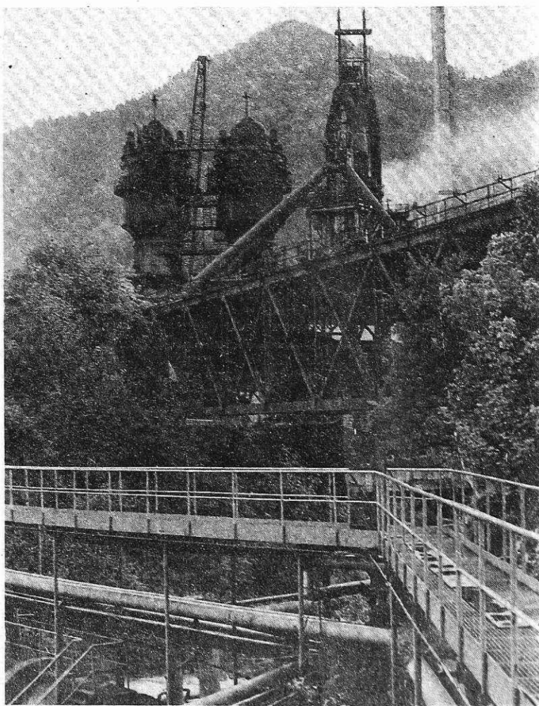
Plinski čistilci na plavžu 2 (foto I. Kučina)
