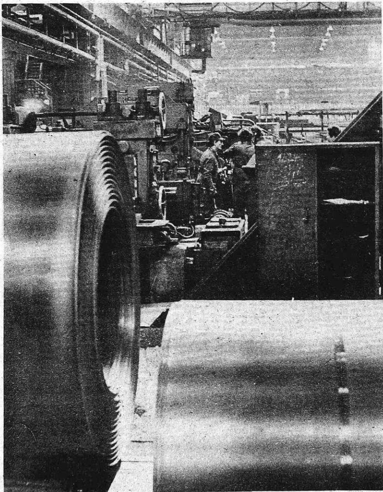
Linija za vzdolžni prerez hladno valjane pločevine (foto I. Kučina)
