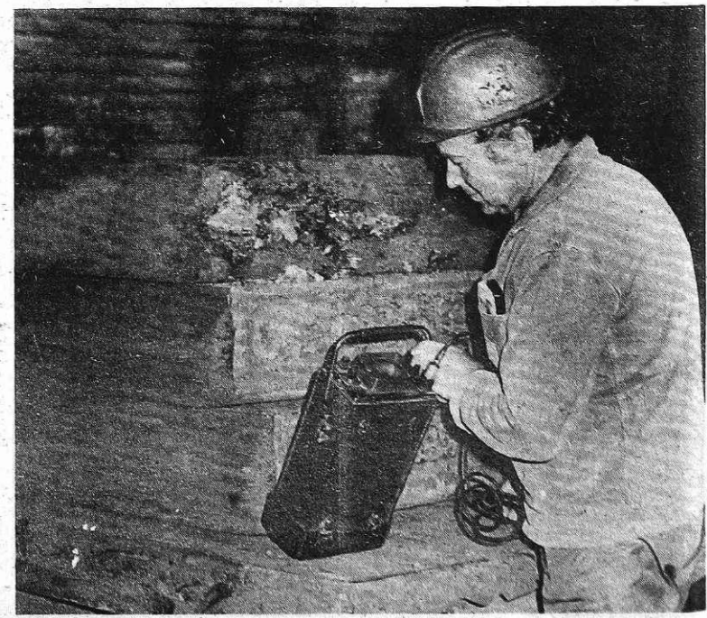
Preizkus slabov z ultrazvokom v valjarni bluming (foto I. Kučina)
