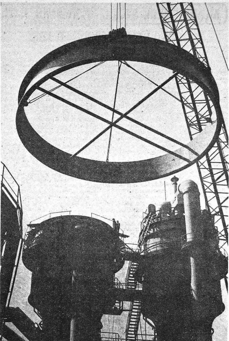
Delavci Hidromontaže nameščajo čistilec na plavžu. Starega je 2. januarja letos razdejala eksplozija plina. Poškodba je bila toliko hujša, ker je bil čistilec že star in razjeden. Dokončanje del pričakujemo te dni (foto S. Kokalj)
