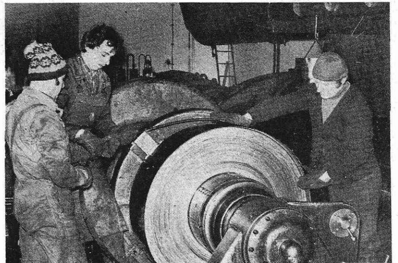
Sodelavci pri Siemag valjarskem stroju v TOZD HVJ
