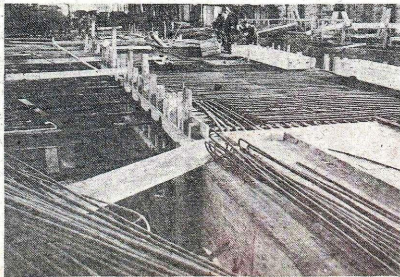
Temelji za novo linijo ravnalnega stroja v TOZD Valjarna debele pločevine (foto I. Kučina)
