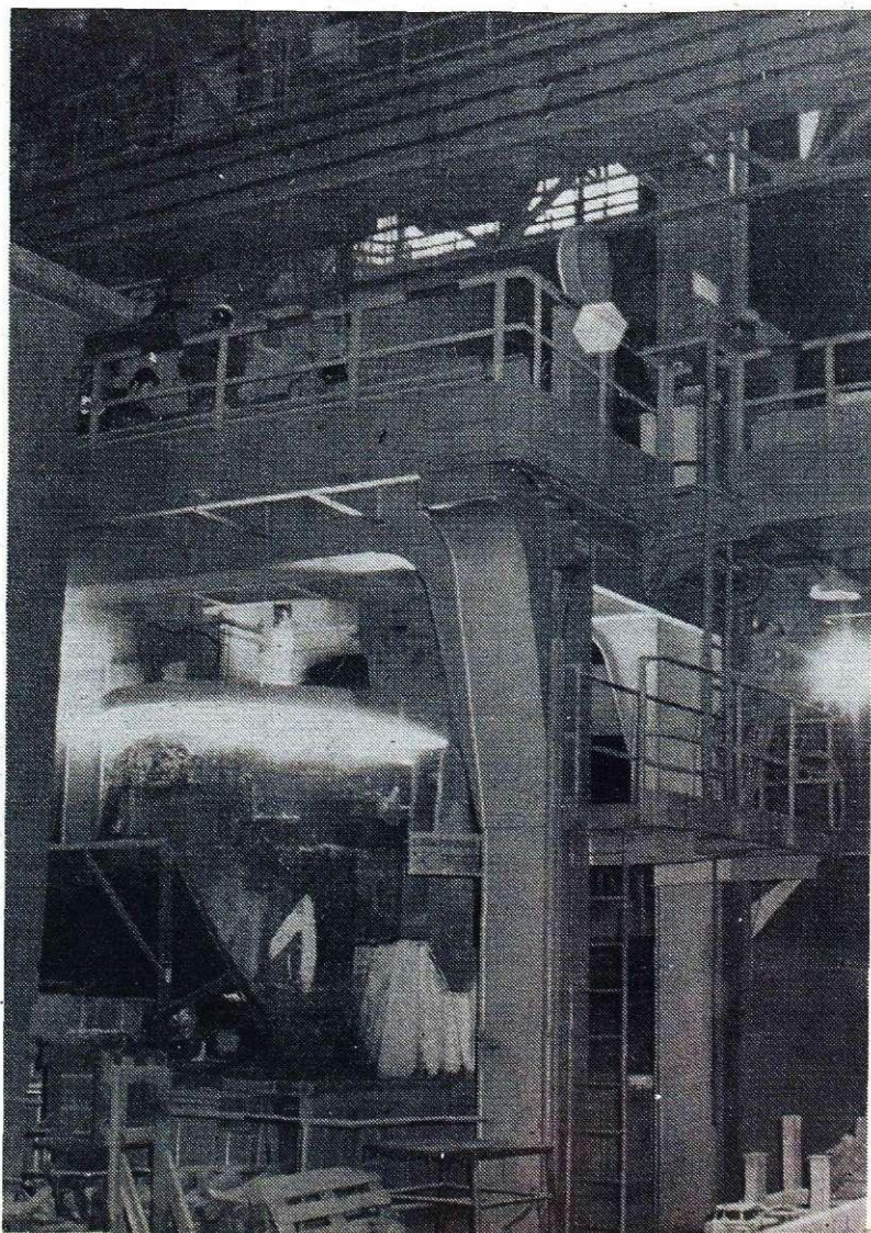
Vpihavanje acetilena v jeklo na konti livu (foto I. Kučina)
