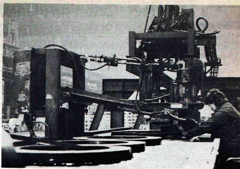
Pakirno-povijalna linija v Hladni valjarni Bela (foto I. Kučina)
