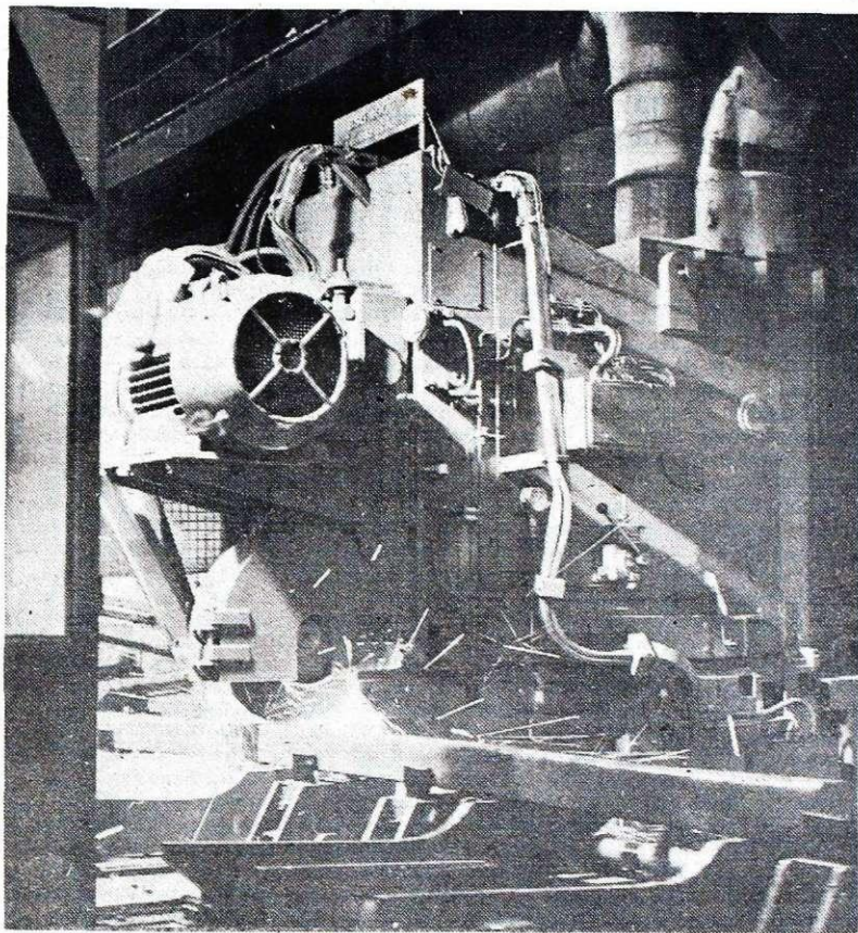
Brusilni stroj BSG 4000 D (foto I. Kučina)
