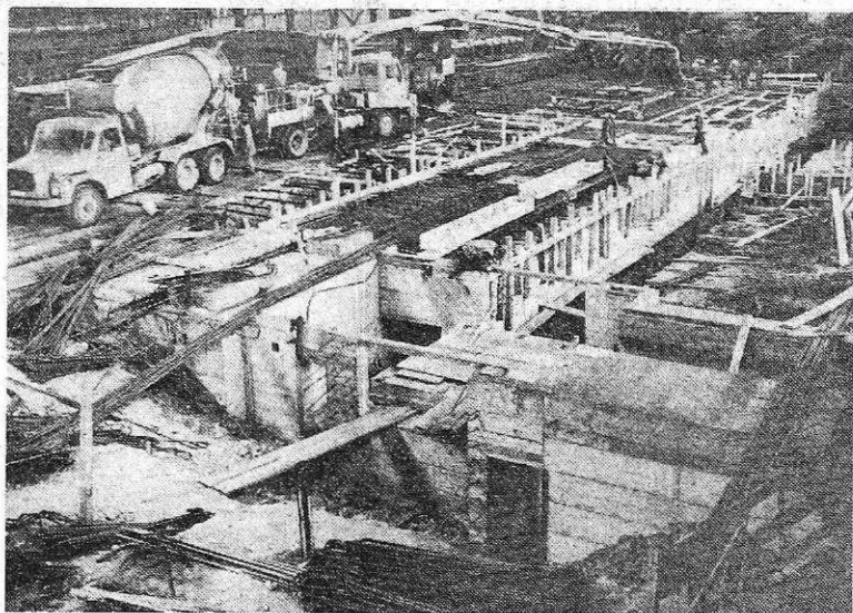
Gradnja temeljev za novo ravnalno linijo v Valjarni debele pločevine (foto I. Kučina)
