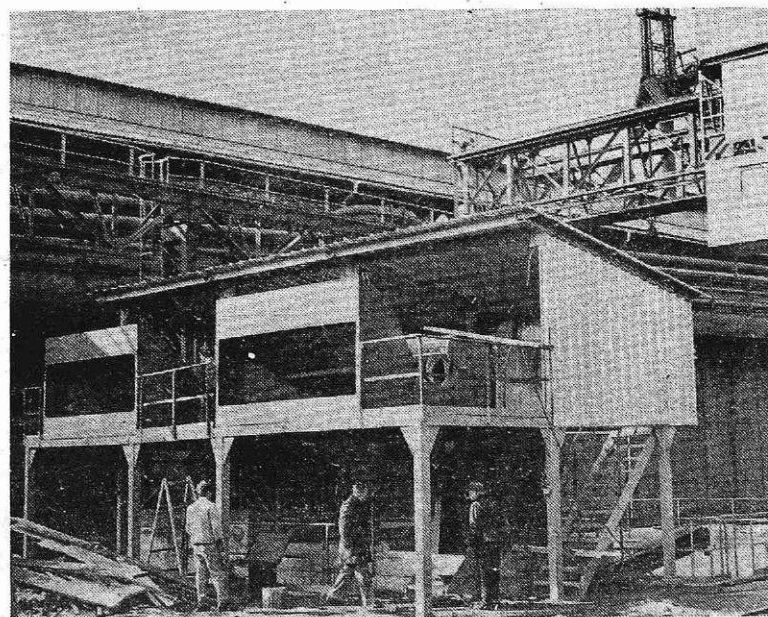
Novi mlin za ostružke že obratuje (foto I. Kučina)
