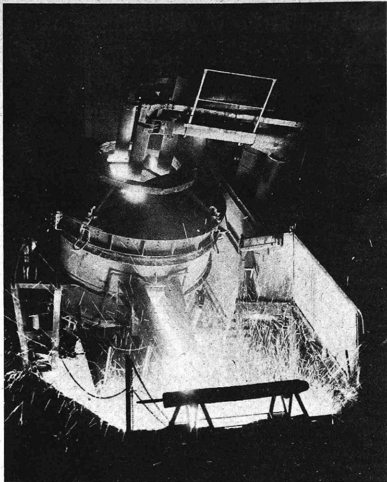
Šarža na BBC električni peči (foto I. Kučina)
