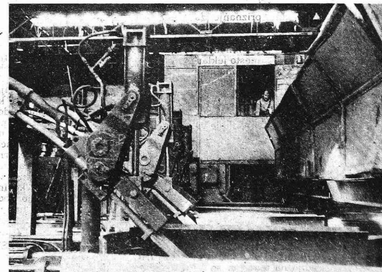
V Valjarni žice in profilov na Beli (foto I. Kučina)
