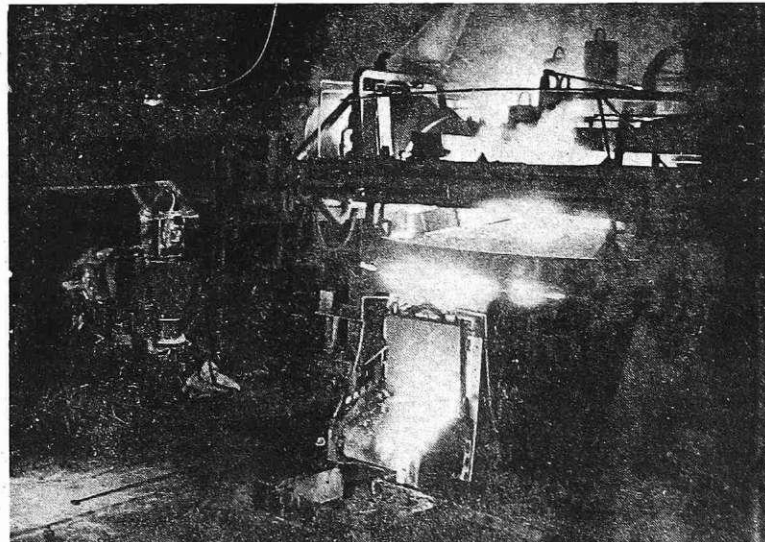
Lectromelt električna peč med obratovanjem (foto I. Kučina)
