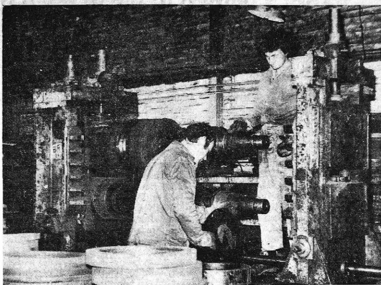
Menjava ogrodja za BRONX škarje v TOZD valjarna bluming stekel (foto I. Kučina)
