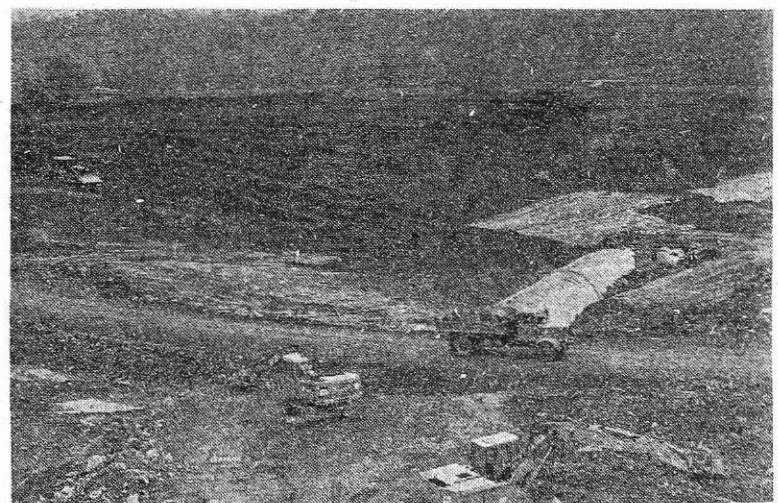
Zemeljska dela za jeklarino 2 (foto I. Kučina)
