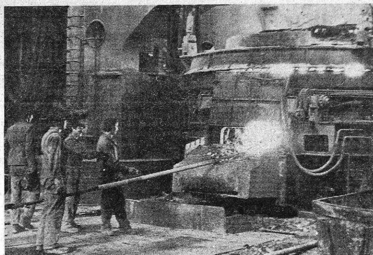
Na dopoldanski dnini v elektrojeklarni (foto I. Kučina)
