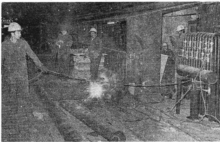
Remont na šesti SM peči (foto I. Kučina)
