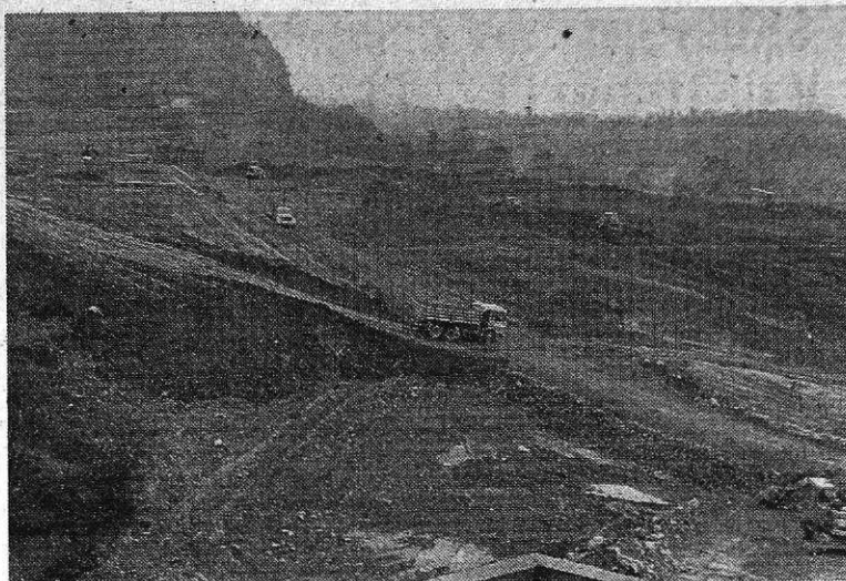
Zemeljska dela za jeklarno 2 (foto I. Kučina)
