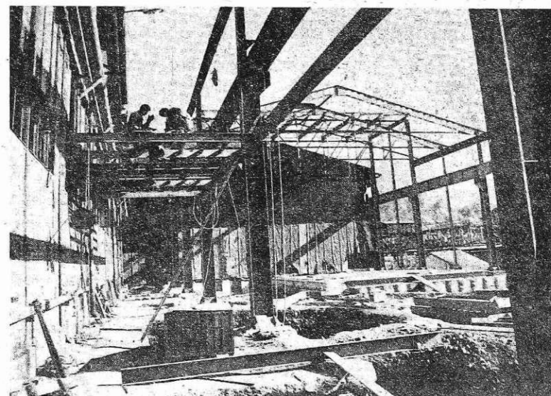
Montaža konstrukcije za novo halo Valjarne debele pločevine (foto I. Kučina)
