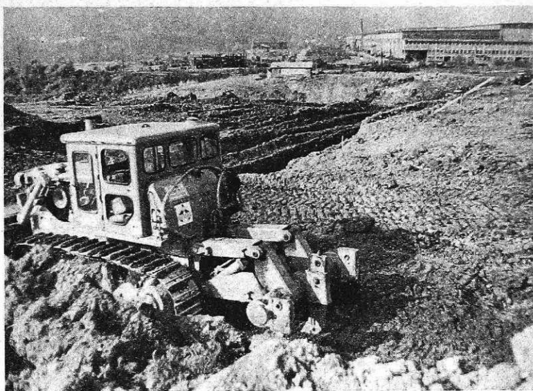
Zemeljska dela za gradnjo jeklarne 2 (foto I. Kučina)
