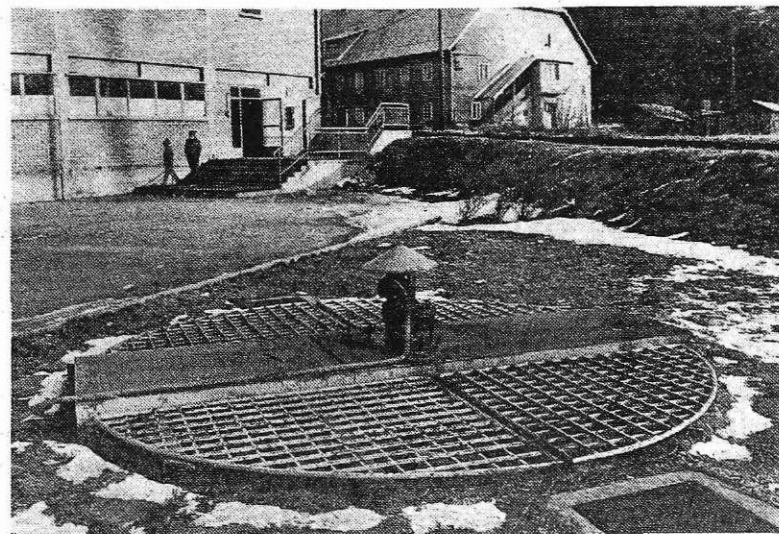
Biološka čistilna naprava v TOZD Vratni podboji
