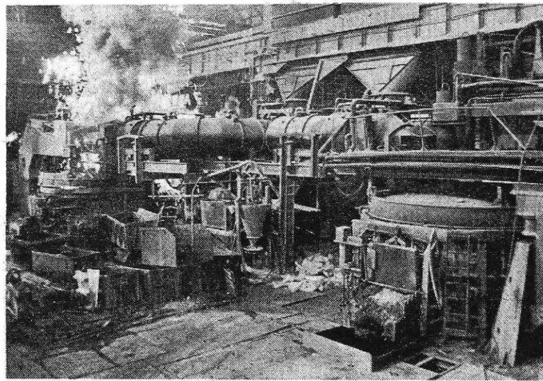
ASEA in LECTROMELT električni peči med obratovanjem (foto I. Kučina)
