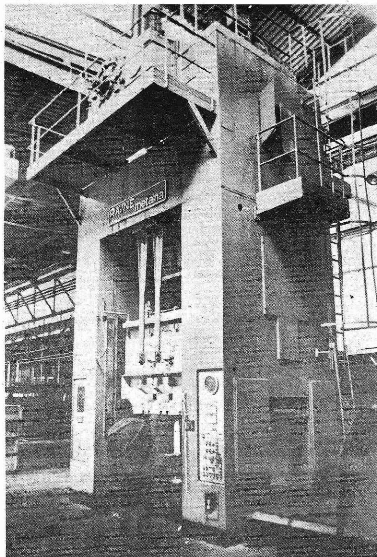
Nova stiskalnica za izdelavo diskov na Javorniku (foto I. Kučina)
