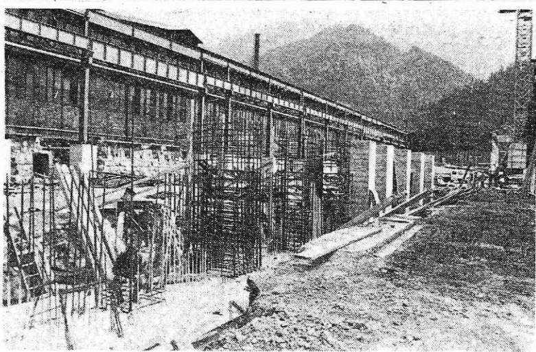
Razširitev hale valjarne debele pločevine (foto I. Kučina)
