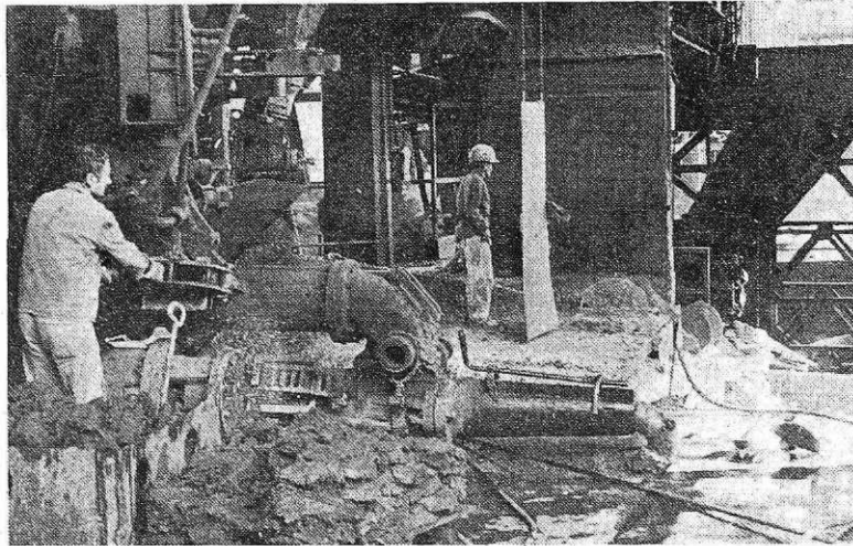
Polnjenje mašilnega stroja z ognjevarno maso na plavžu (foto I. Kučina)
