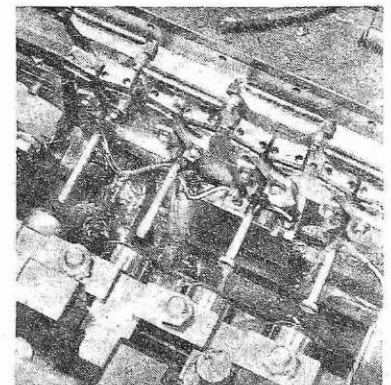
Rezanje, prenos in preoblikovanje v štirih matricah
