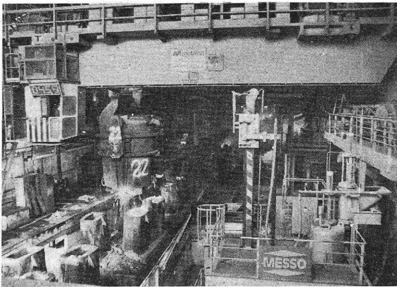
Vlivanje jekla, desno vakuumška naprava (foto I. Kučina)
