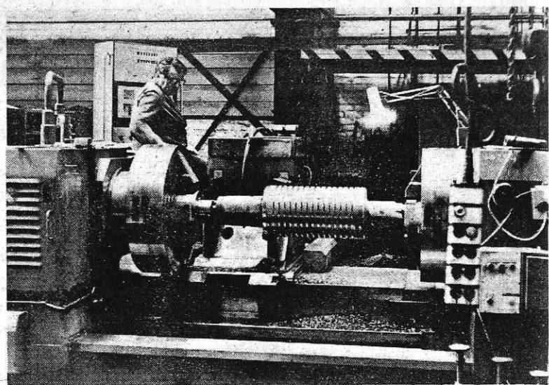
V strugarni valjev na Beli (foto I. Kučina)
