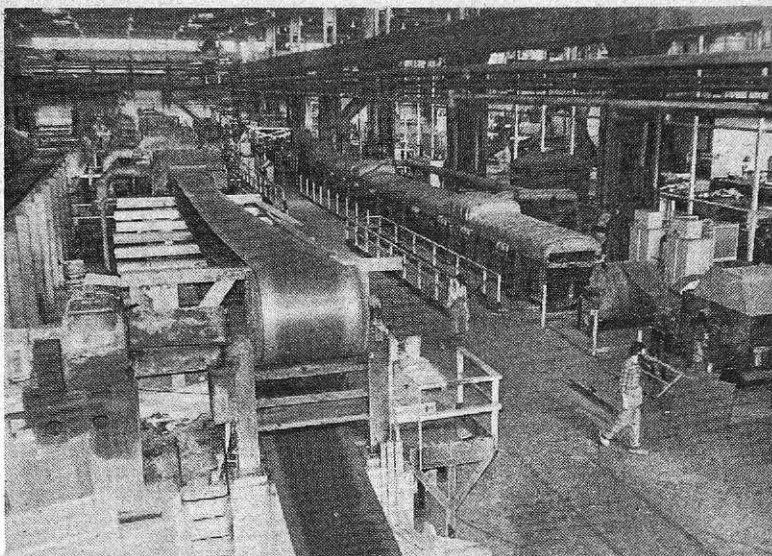
Lužilno-žarilna linija v hladni valjarni Bela (foto I. Kučina)
