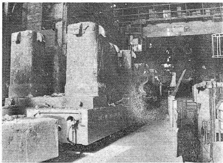
Kokile na poti v jeklarno (foto I. Kučina)
