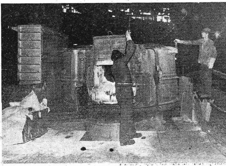
Pri BBC električni peči (foto I. Kučina)
