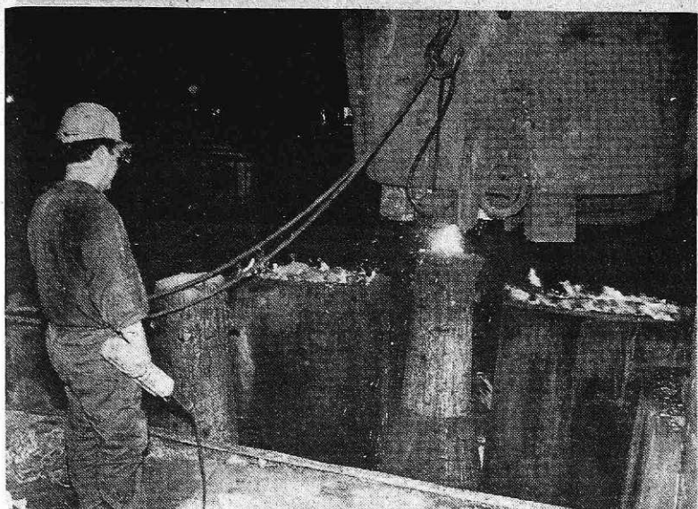
Vlivanje jekla (foto I. Kučina)
