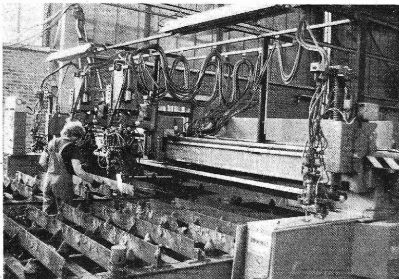
Delo na sektorju v obratu OTOP v novem prizidku valjarne debele pločevine (foto S. Kokalj)
