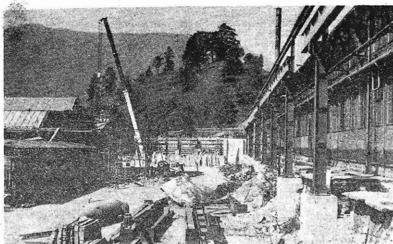
Priprava temeljev za gradnjo prizidka Valjane debele pločvine
