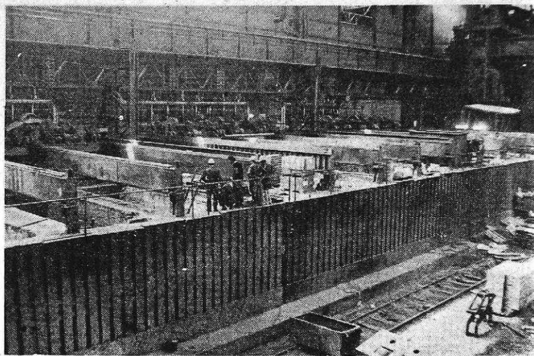
Pogled na globinske peči v valjarni bluming med remontom (foto S. Kokalj)
