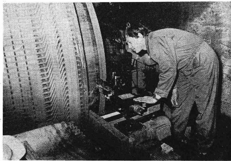
Struženje elektro motorja v strojnici valjarne bluming (foto S. Kokalj)
