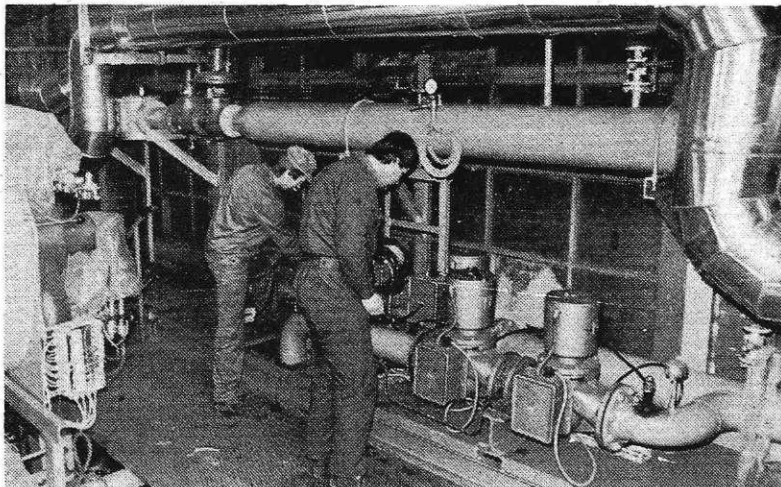
Gorilnik Klöckner v zaključni fazi montaže na vročevodnem kotlu na Jesenicah (foto I. Kučina)
