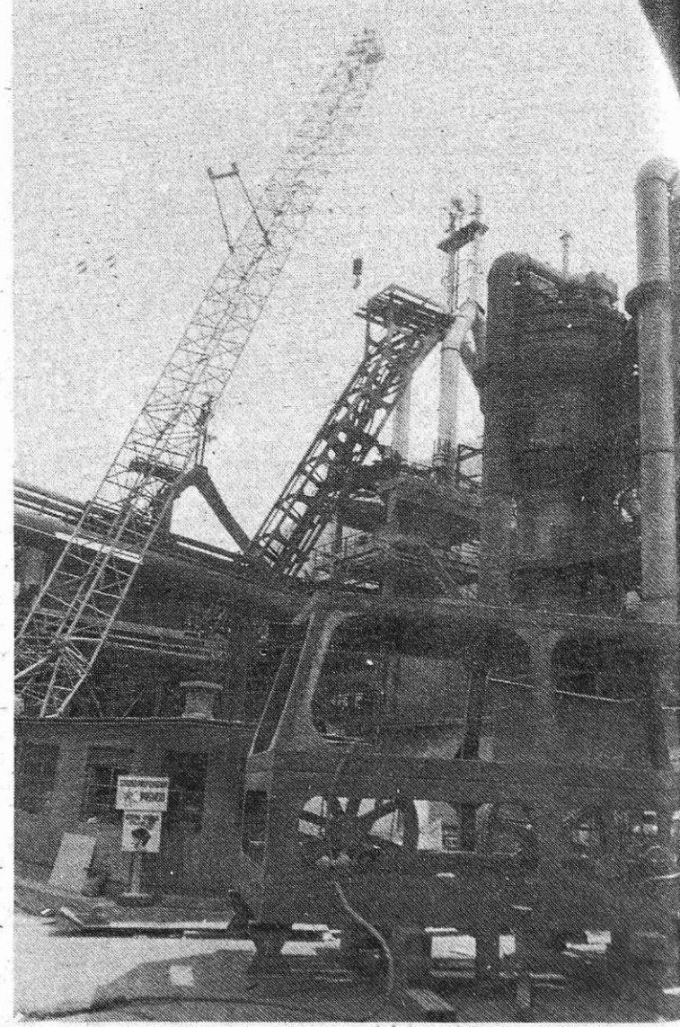
Montaža poševnega dvigala na plavžu (foto S. Kokalj)
