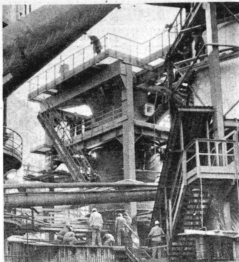
Montaža plavža 2 (foto I. Kučina)
