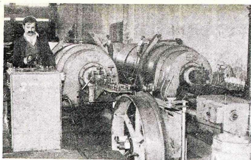
Pletilnica žice v TOZD Žičarna (foto I. Kučina)
