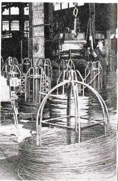
Patentirnica v TOZD Žičarna (foto I. Kučina)
