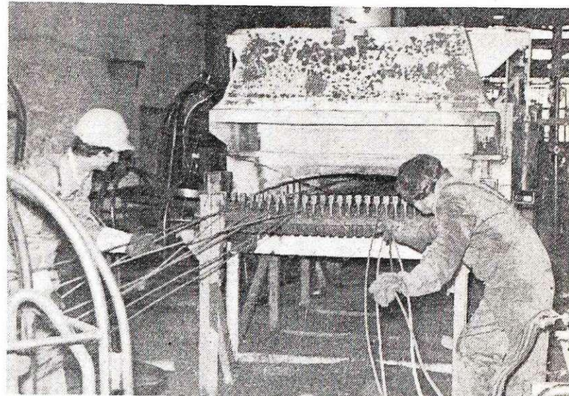
Žarilna peč v patentirnici TOZD Žičarna (foto I. Kučina)
