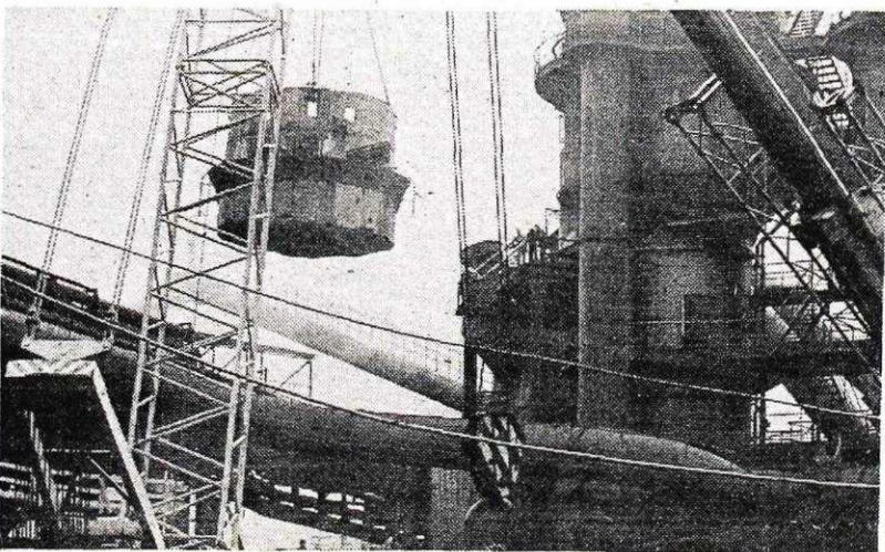
Med remontom plavža 2 (foto B. Grce)
