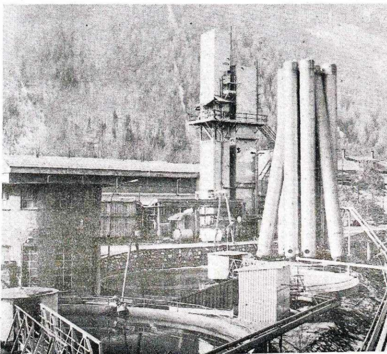
Kisikarna »Sava« (foto S. Kokalj)
