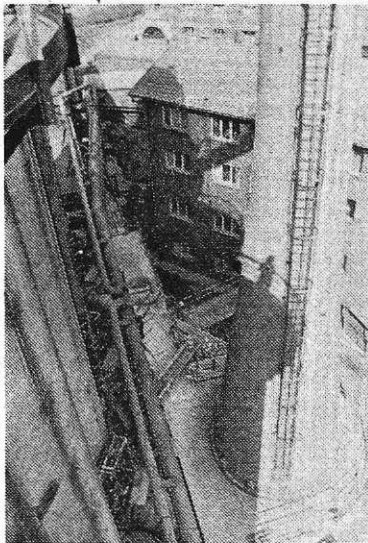
Remontna dela na kavperjih (foto I. Kučina)
